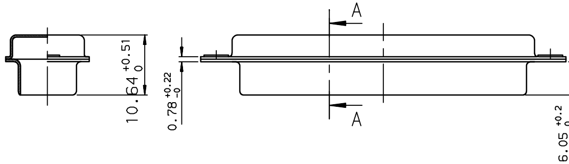
1/2 COUPE A-A
